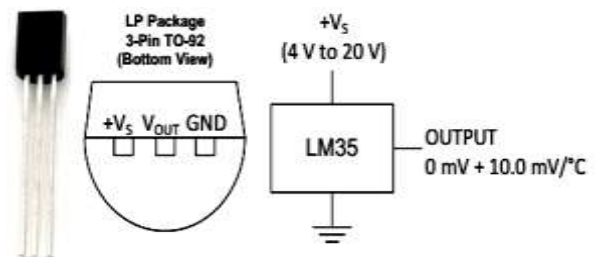
Gambar 4. LM35
