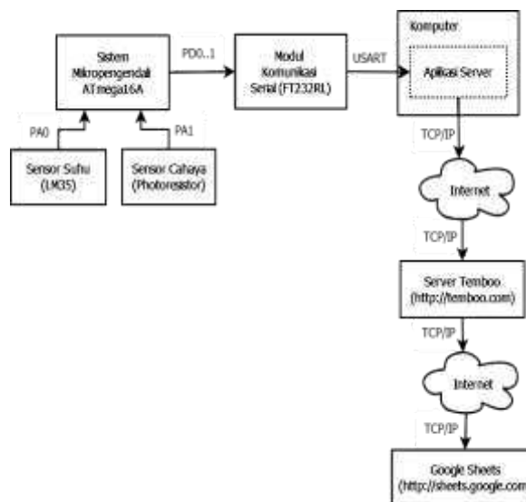
Gambar 6. Sistem Keseluruhan
