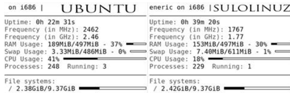
Gambar 5. Perbandingan Load CPU dan RAM usage pada saat melakukan pemantauan kinerja jaringan
