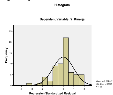
Gambar 2. Uji Normalitas
