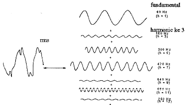
Gambar 1. Bentuk gelombang harmonisa dengan frekuensi dasar 60 Hz
