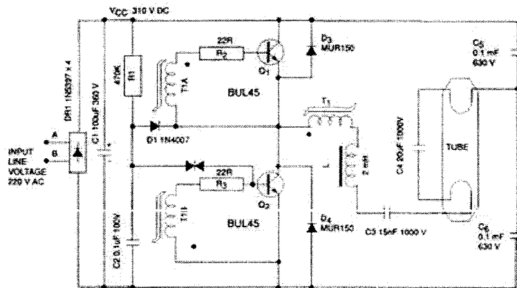
Gambar 4. Rangkaian balast elektronik
