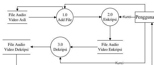
Gambar 5. DAD Level 0 (Overview)
