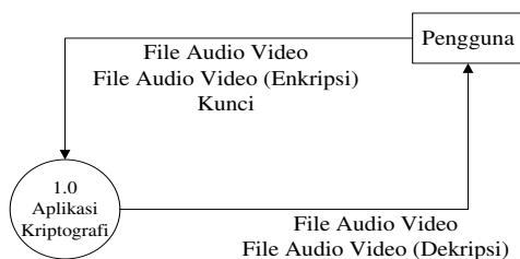
Gambar 4. Diagram Konteks
