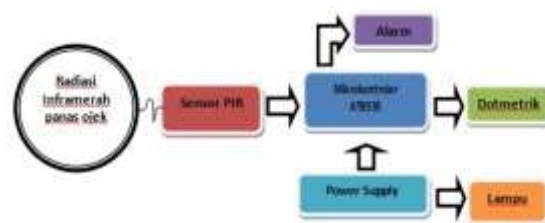
Gambar 5. Perancangan Rangkaian Sistem Mikrokontroller ATMEGA8535
