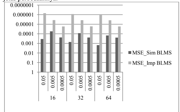
Gambar 14 Perbandingan MSE simulasi dan Implementasi algoritma BLMS
