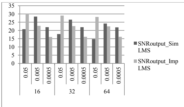
Gambar 13 Perbandingan SNR simulasi dan Implementasi algoritma LMS
