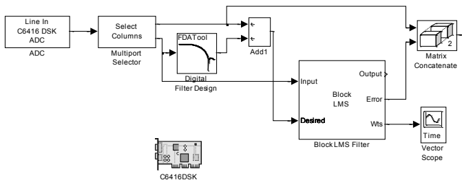
Gambar 4 Rangkaian blok Implementasi Sistem Multiport
