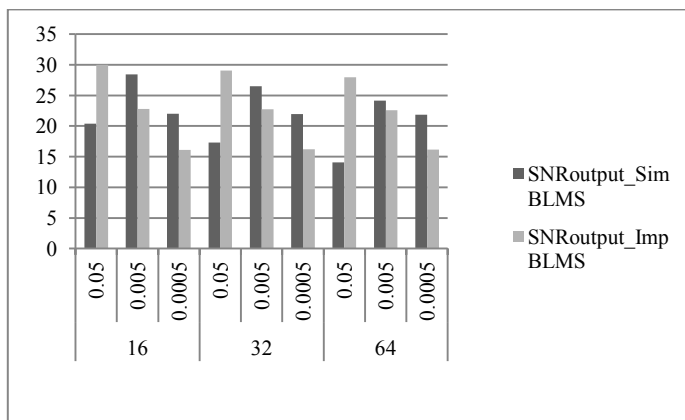
Gambar 12 Perbandingan SNR simulasi dan Implementasi algoritma BLMS
