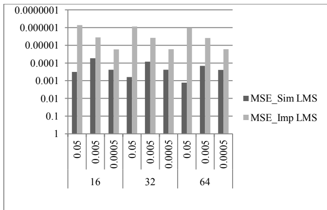
Gambar 15 Grafik perbandingan nilai MSE simulasi dengan implementasi algoritma LMS
