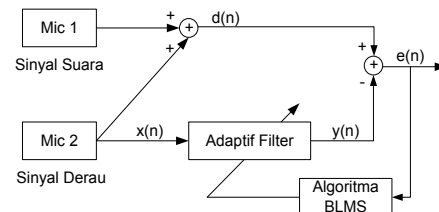
Gambar 2 Diagram Blok Sistem
