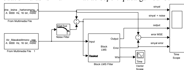
Gambar 3 Diagram Blok Simulasi filter adaptif BLMS
