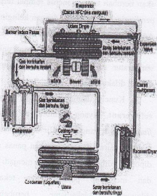
Gambar 1. Siklus kerja AC
