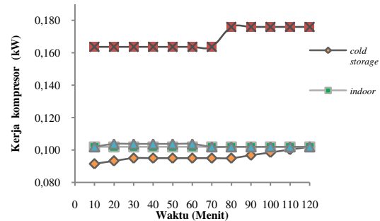
Gambar 4. Grafik perbandingan kerja kompresi terhadap waktu
