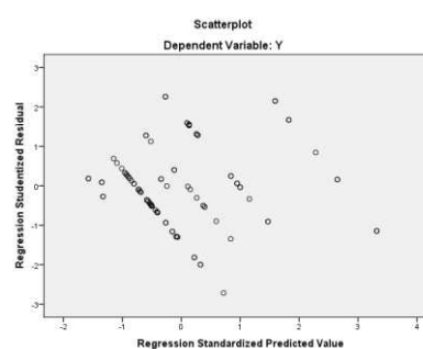
Gambar 2, Uji Heteroskedastisitas
