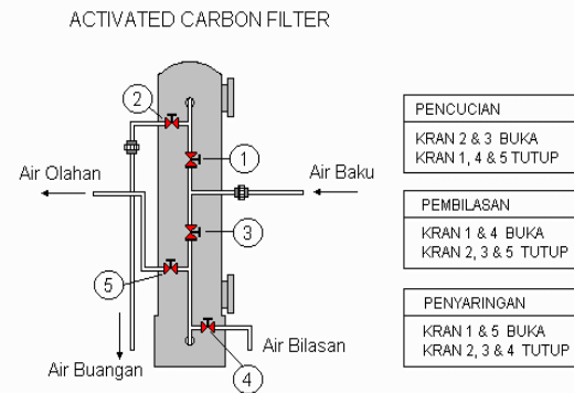
Gambar 5 : Skema pengoperasian filter karbon aktif.
