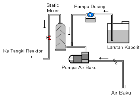
Gambar 1 : Skema injeksi larutan Kaporit.
