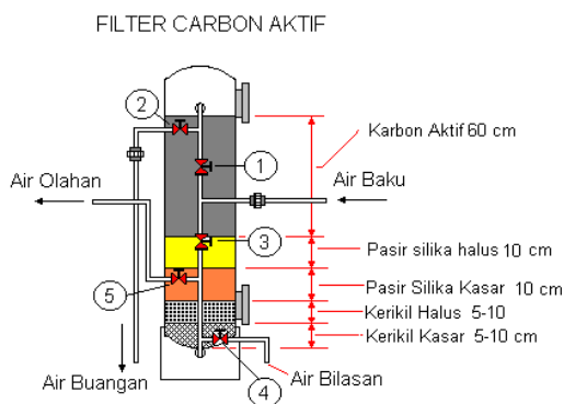
Gambar 4 : Susunan media di dalam filter karbon aktif.
