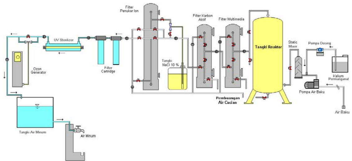
Gambar 7 : Diagram proses pengolahan air sadah menjadi air siap mnum.
