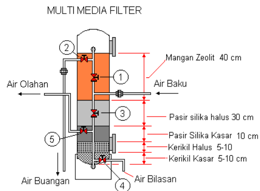
Gambar 2 : Susunan media di dalam filter multi-media.
