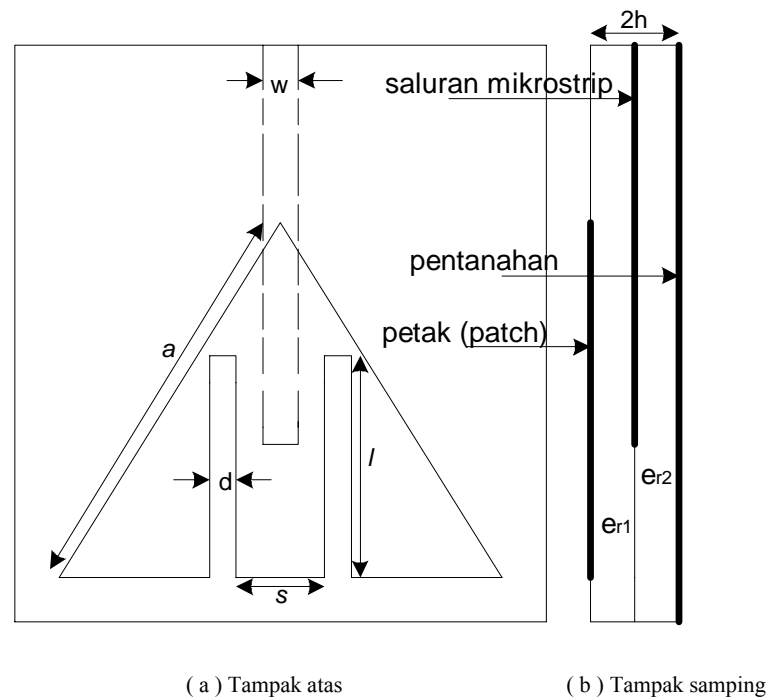
Gambar 3. Geometri antenna rancangan dengan sepaang celah menggunakan saluran mikrostrip
