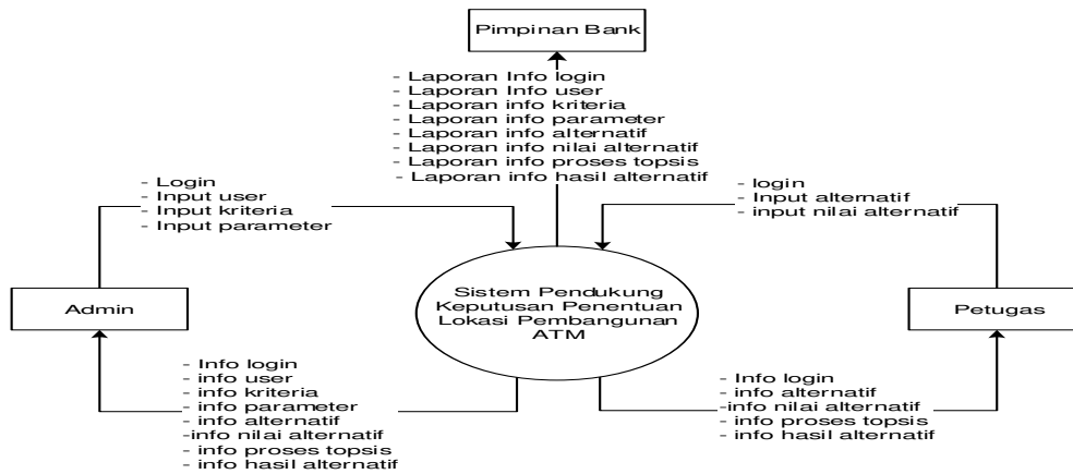
Gambar 4 Konteks Diagram
