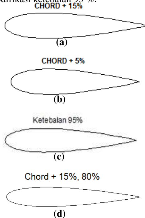
Gambar 13. Perbandingan Geometri foil yang Memiliki Performa Terbaik, a)Foil dengan Rasio C_L / C_D Paling Besar. b)Foil dengan Torsi Terbesar untuk Panjang Chord. c)Foil dengan Torsi Terbesar untuk Ketebalan. d)Foil dengan Torsi Terbesar untuk Kombinasi
