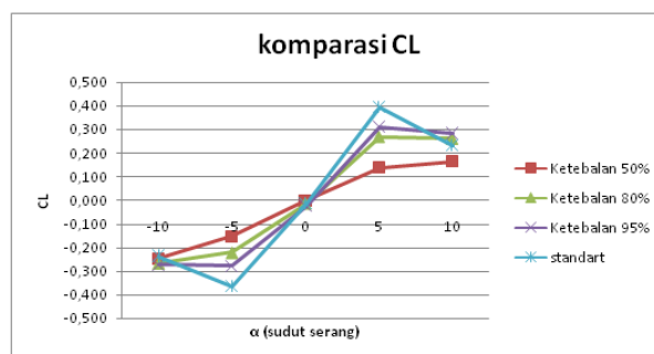
Gambar 2. Hasil Simulasi Numerik Modifikasi untuk C_L
