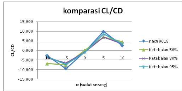
Gambar 6. Grafik Nilai C_L/C_D untuk Modifikasi Ketebalan
