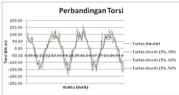
Gambar 11. Perbandingan Torsi pada Turbin Standart dengan Turbin Modifikasi kombinasi panjang chord 15% dengan ketebalan 95%, 80%, dan 50%
