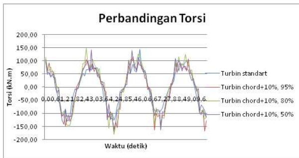
Gambar 12. Perbandingan Torsi pada Turbin Standart dengan Turbin Modifikasi kombinasi panjang chord 10% dengan ketebalan 95%, 80%, dan 50%
