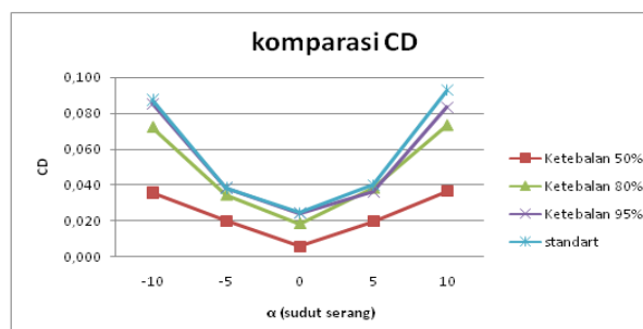
Gambar 3. Hasil Simulasi Numerik Modifikasi untuk C_D
