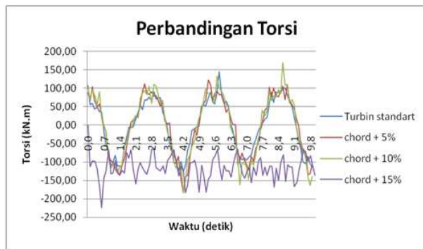
Gambar 8. Perbandingan Torsi pada Turbin Standart dengan Turbin Modifikasi Panjang Chord
