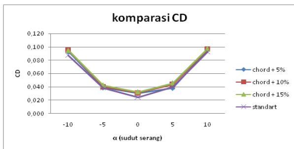
Gambar 5. Hasil Simulasi Numerik Modifikasi untuk C_D
