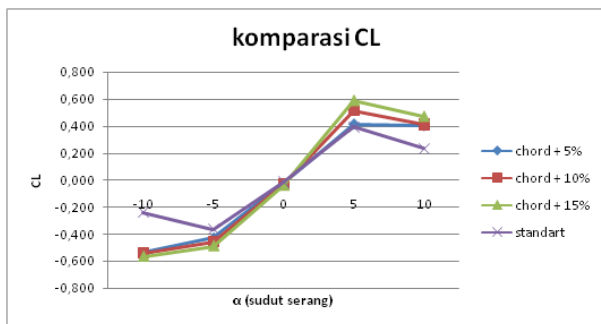
Gambar 4. Hasil Simulasi Numerik Modifikasi untuk C_L
