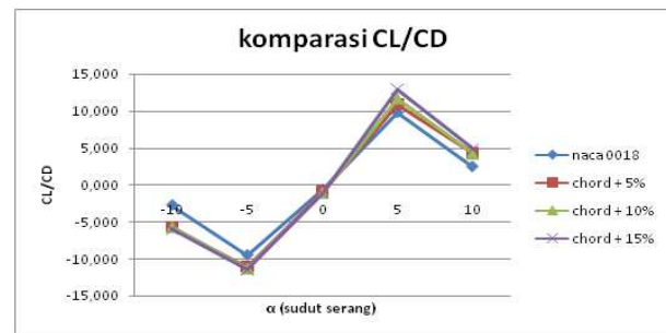
Gambar 7. Grafik Nilai C_L/C_D untuk Modifikasi Panjang Chord
