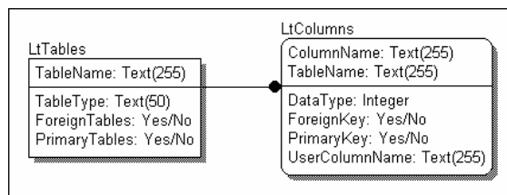
Gambar 8. ERD Struktur Database OLAP Report.
