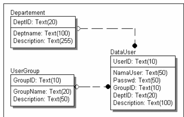
Gambar 6. Hubungan Tabel-Tabel dalam User Management.
