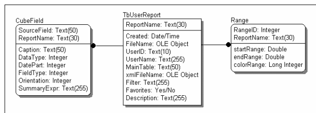
Gambar 9. ERD Penyimpanan Display Analisis OLAP Report.
