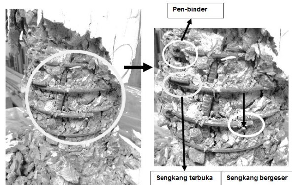
Gambar 10. Detail kegagalan tulangan pengekan tidak standar dengan perkuatan pen-binder
