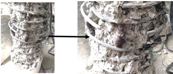
Gambar 8. Detail kegagalan tulangan pengekan standar/spiral
