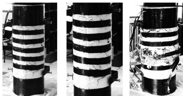
Gambar 11. Pola retak benda uji kolom lingkaran tulangan pengekan tidak standar dengan perkuatan FRP
