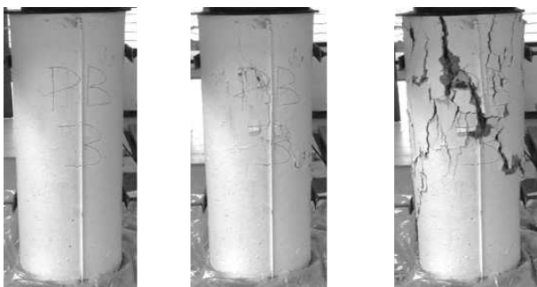
Gambar 9. Pola retak benda uji kolom lingkaran tulangan pengekan tidak standar dengan perkuatan pen-binder
