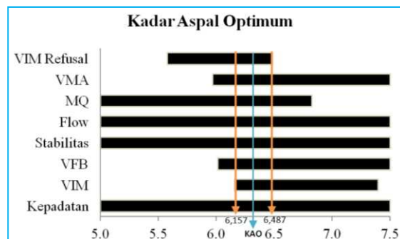
Gambar 4 Kadar Aspal Optimum untuk Campuran AC-BC pada Kadar Kapur 25 %
