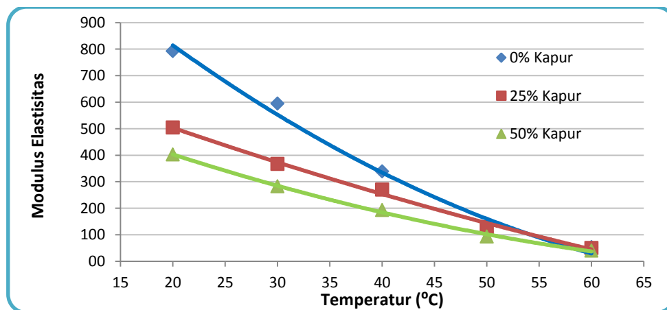
Gambar 8 Hubungan antara Temperatur terhadap Modulus Elastisitas
