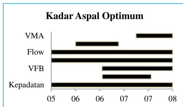
Gambar 6 Kadar Aspal Optimum untuk Campuran AC-WC pada Kadar Kapur 75 %
