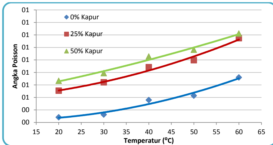
Gambar 10 Hubungan antara Temperatur dan Angka Poisson
