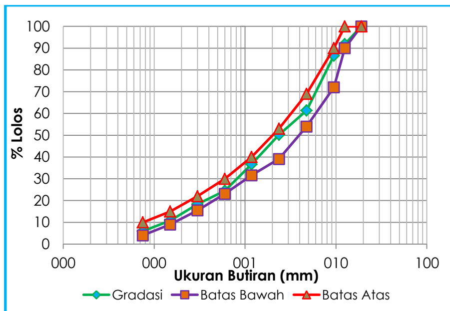
Gambar 2 Gradasi Gabungan Campuran Beton Aspal Lapis Aus
