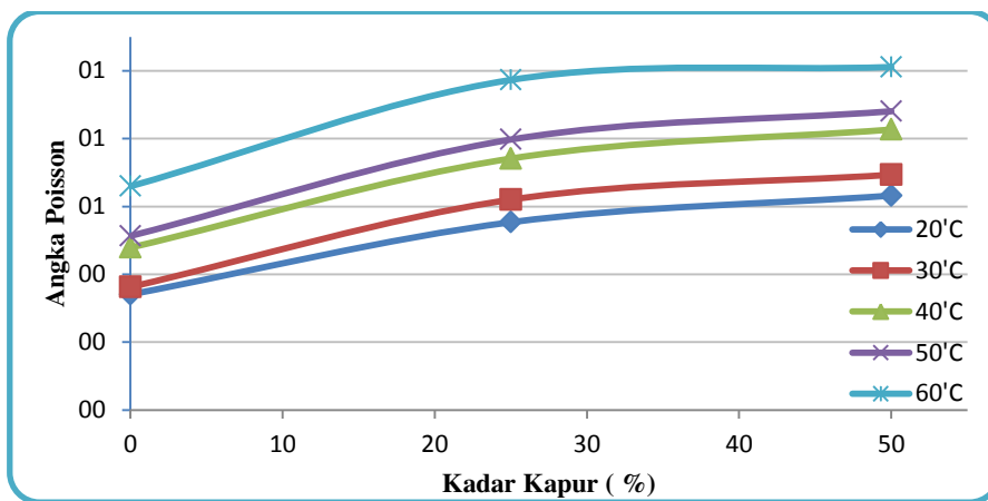
Gambar 11 Hubungan antara Kadar Kapur dan Angka Poisson
