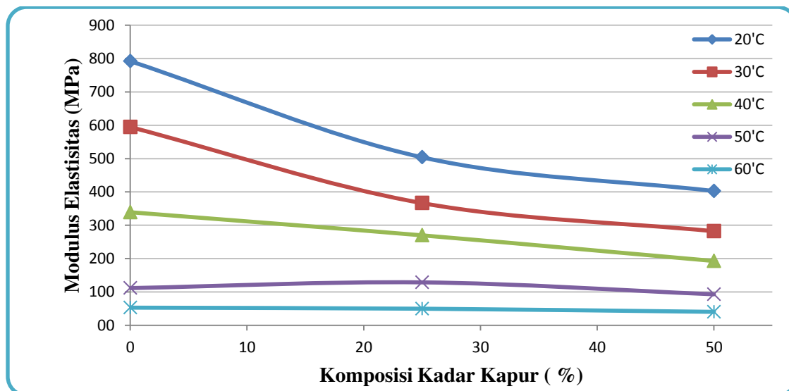
Gambar 9 Hubungan antara Komposisi Kadar Kapur terhadap Modulus Elastisitas
