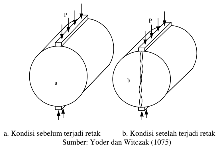
Gambar 1 Pengujian Kuat Tarik Tidak Langsung
