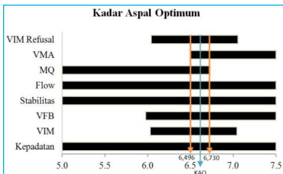
Gambar 5 Kadar Aspal Optimum untuk Campuran AC-WC pada Kadar Kapur 50 %
