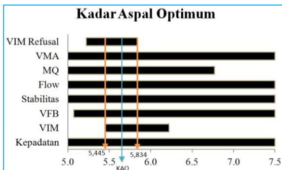
Gambar 3 Kadar Aspal Optimum untuk Campuran AC-WC pada Kadar Kapur 0 %
