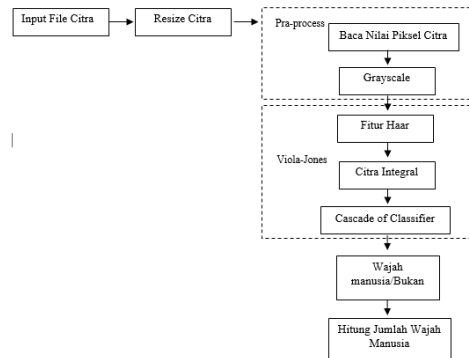
Gambar 1. Arsitektur Umum
