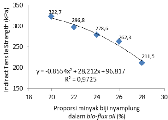
Gambar 15. Nilai ITS pada kadar aspal optimum
