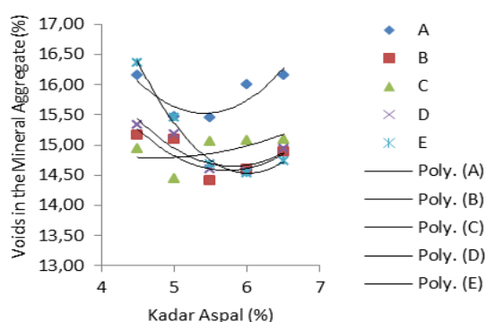
Gambar 7. Kadar aspal vs VMA
