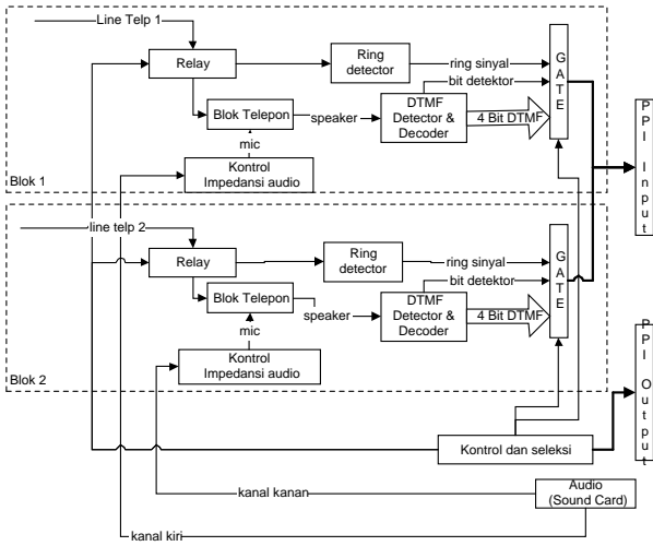
Gambar 5. Bagan rangkaian penerima DTMF
