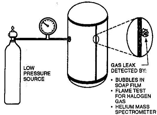
Gambar 13. Uji Kebocoran
