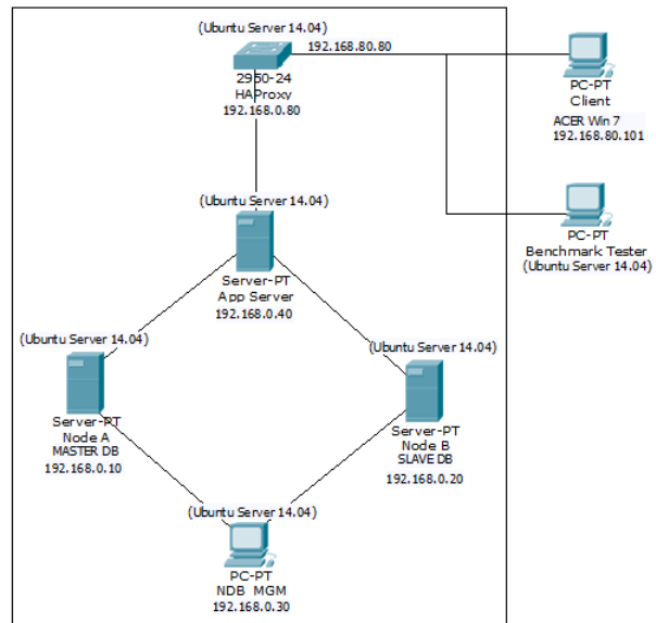
Gambar 1 Topologi Sistem
