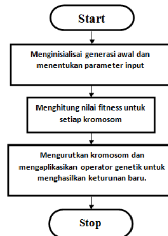
Gambar. 3. flowchart optimasi batas interval menggunakan Algoritma genetic.
