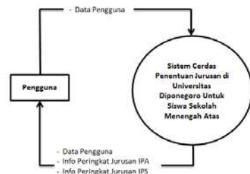
Gambar 2 Diagram Konteks
