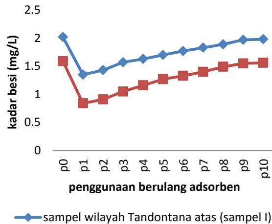
Gambar 2. Kurva hubungan antara penggunaan berulang adsorben dengan kadar besi pada air sumur.
