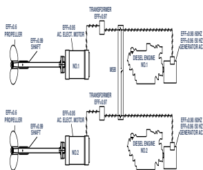
Gambar 5.5. Efisiensi pada DEP
