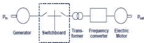
Gambar 5.4. Skema propulsi listrik
