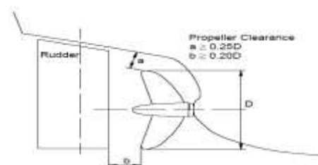
Gambar 5.3. Batasan propeler pada kapal
