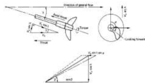
Gambar 2 – Gaya Trust yang bekerja pada kapal cepat
