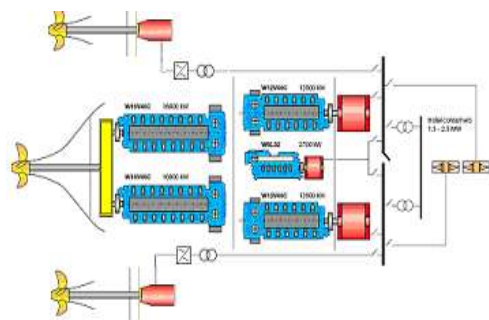
Gambar 5.7. Aplikasi instalasi hybrid (DMP&DEP) propulsi
