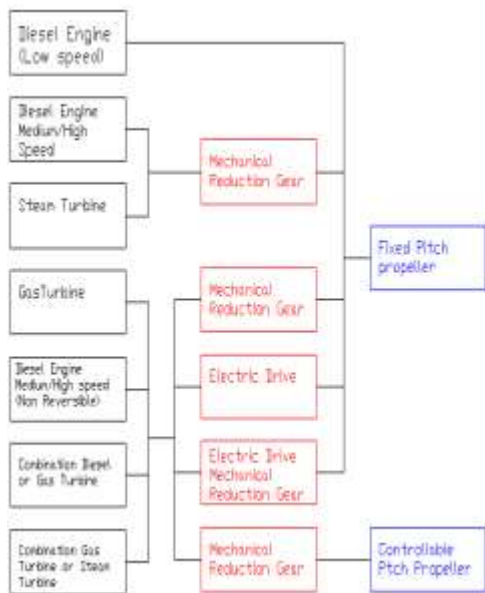
Gambar 5.1. Konfigurasi sistem propulsi di kapal
