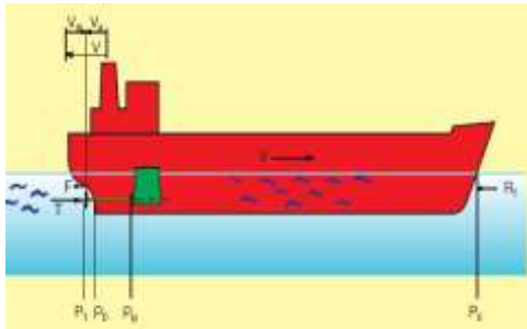
Gambar 5.8 Gaya-gaya yang bekerja pada sistem penggerak kapal
