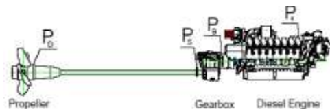
Gambar 5.9 Daya pada sistem penggerak dikapal
