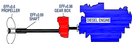
Gambar 5.6. Efisiensi pada DMP
