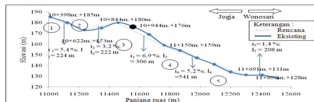
Gambar 2 Penampang Memanjang Ruas Jalan Yogyakarta – Wonosari di Bunder
