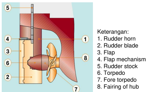
Gambar.3. Perpaduan propeller dan rudder
