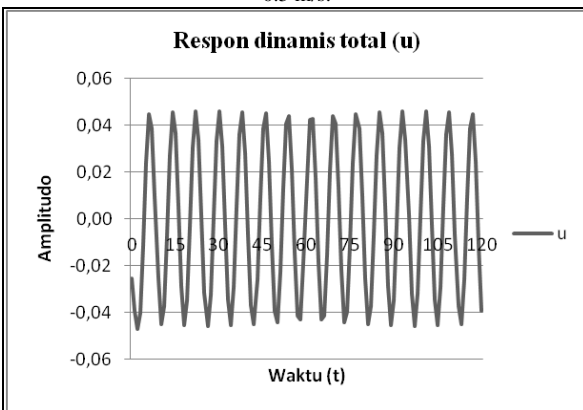
Gambar 12. Grafik amplitudo yang dihasilkan model II pada kecepatan awal 0,5 m/s.
