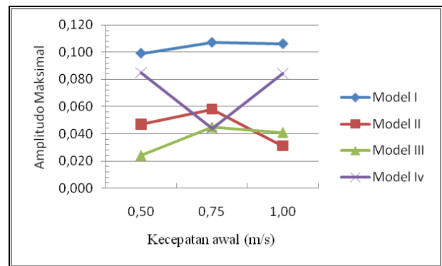
Gambar 15. Grafik nilai amplitudo maksimum
