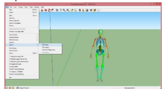
Gambar 9 Ekspor Objek
