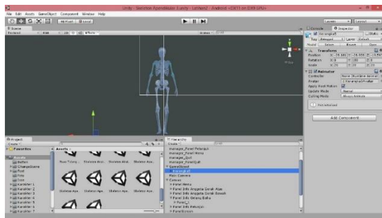
Gambar 11 Inspektor Objek
