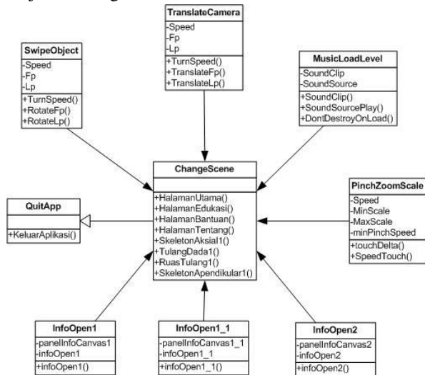
Gambar 8 Diagram Kelas
