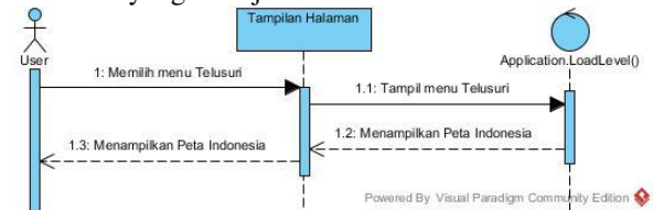
Gambar 3. Sequence diagram memilih menu Telusuri
