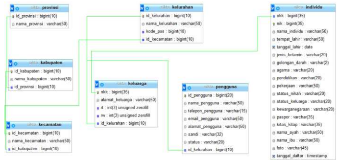
Gambar 5 Relasi Tabel
