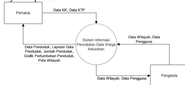
Gambar 2 Diagram Konteks
