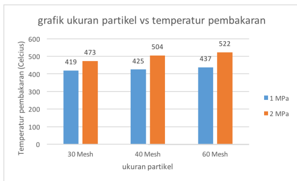
Gambar 9 Pengaruh ukuran partikel terhadap temperatur pembakaran
