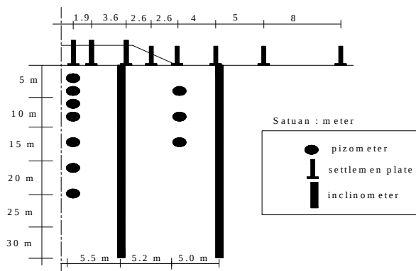
Gambar 3. Posisi instrumen geoteknik di lapangan (Balai Geoteknik Jalan, 2002)
