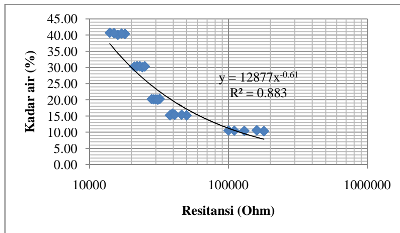
Gambar 10. Hubungan Resistansi dan Kadar Air Tanah
