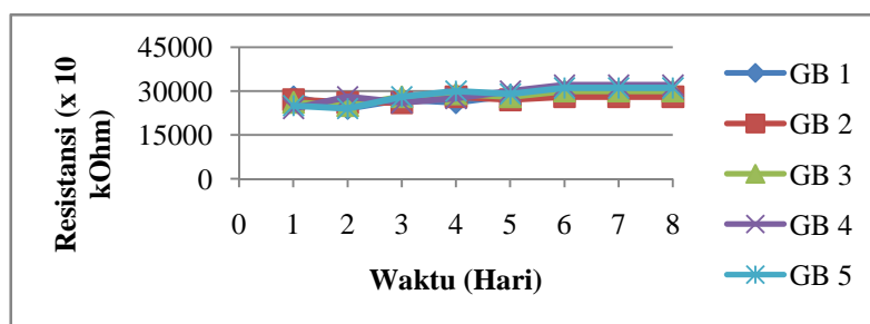
Gambar 7. Pembacaan Resistansi Kadar Air Tanah 20 %
