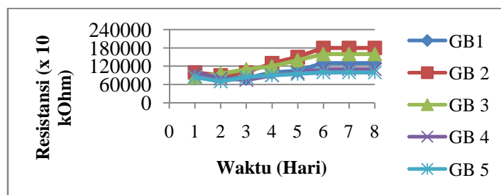
Gambar 5. Pembacaan Resistansi Kadar Air Tanah 10
