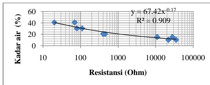
Gambar 1. Nilai Resistansi dengan Kadar Air Tanah Lempung Sumber: Sir, 2010.
