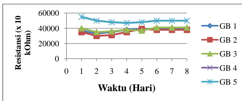
Gambar 6. Pembacaan Resistansi Kadar Air Tanah 15 %
