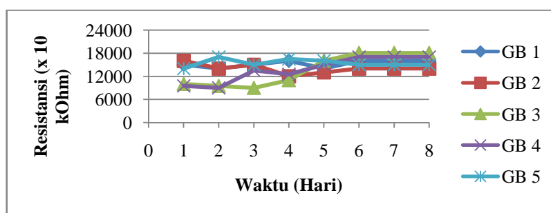
Gambar 9. Pembacaan Resistansi Kadar Air Tanah 40 %
