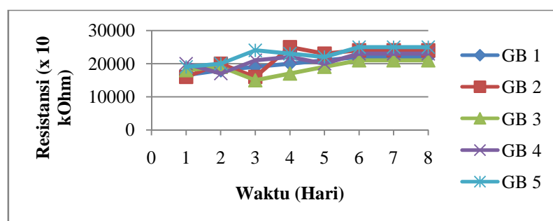
Gambar 8. Pembacaan Resistansi Kadar Air Tanah 30 %
