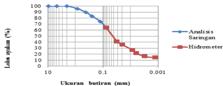
Gambar 4. Analisa Distribusi Ukuran Butiran
