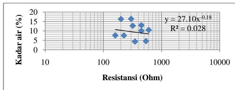
Gambar 2. Nilai Resistansi dengan Kadar Air Tanah Pasir Sumber: Sir, 2010.
