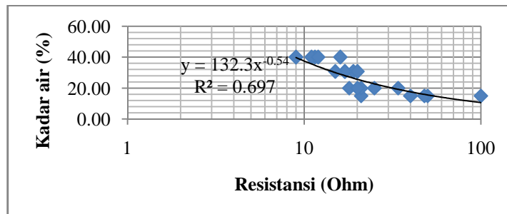
Gambar 3. Hubungan Resistansi dengan Kadar Air Tanah Lempung (Nesnay, 2012)
