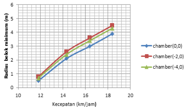
Gambar 6. Kurva Hubungan antara Kecepatan dan Kemampuan Belok Mobil 4WD
