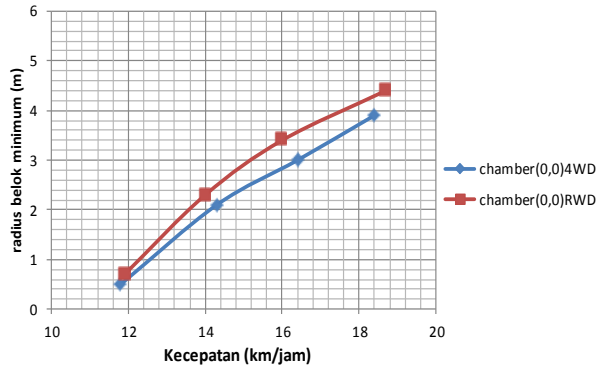
Gambar 9. Kurva Kemampuan Belok Mobil RWD & 4WD dengan Camber 0^{\circ}
