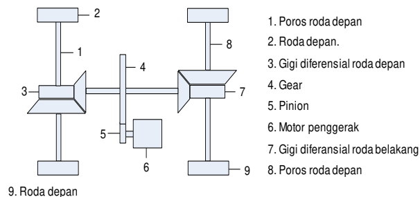
Gambar 1. Sistem Penggerak Mobil Uji
