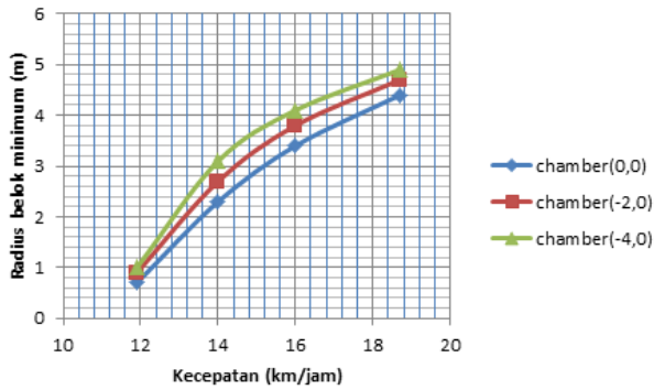
Gambar 7. Kurva Hubungan antara Kecepatan dan Kemampuan Belok Mobil RWD
