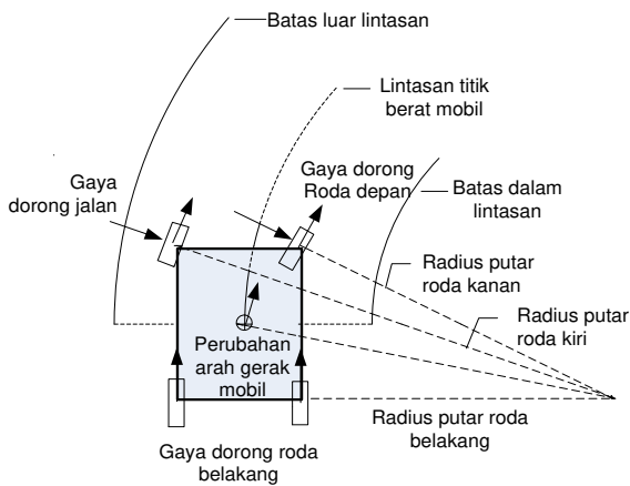
Gambar 8. Diagram Gaya pada Mobil
