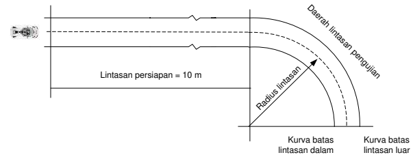
Gambar 3. Lintasan uji
