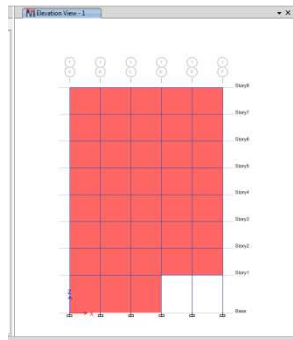
Gambar 4. Struktur Dengan 60% Dinding Pengisi Pada Lantai Dasar
