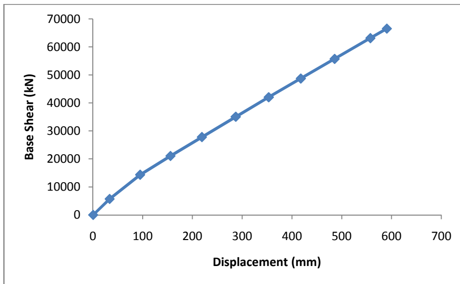
Gambar 16. Kurva Kapasitas Pada Spesimen Dengan 80 % Dinding Pengisi Pada Lantai Dasar
