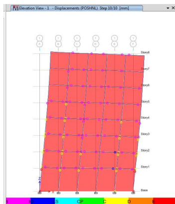
Gambar 17. Hasil Analisis Pushover Pada Struktur Gedung Dengan 100% Dinding Pengisi Pada Lantai Dasar.
