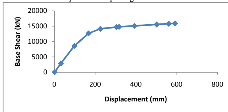
Gambar 10. Kurva Kapasitas Pada Struktur Dengan 20% Dinding Pengisi Pada Lantai Dasar
