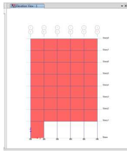
Gambar 2. Struktur Dengan 20% Dinding Pengisi Pada Lantai Dasar
