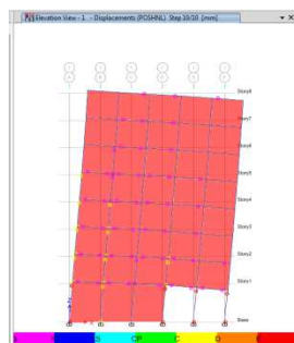
Gambar 13. Hasil Analisis Pushover Pada Struktur Gedung Dengan 60% Dinding Pengisi
