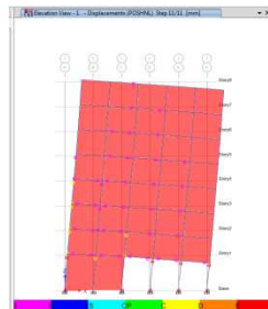
Gambar 11. Hasil Analisis Pushover Pada Struktur Gedung Dengan 40% Dinding Pengisi Pada Lantai Dasar.
