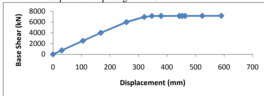
Gambar 8. Kurva Kapasitas Pada Struktur Tanpa Dinding Pengisi Pada Lantai Dasar
