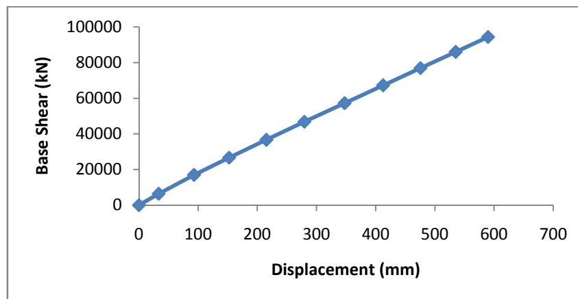
Gambar 18. Kurva Kapasitas Pada Struktur Dengan 100 % Dinding Pengisi Pada Lantai Dasar
