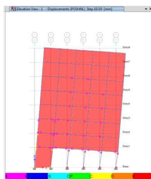
Gambar 9. Hasil analisis pushover pada struktur dengan 20% dinding pengisi pada lantai dasar
