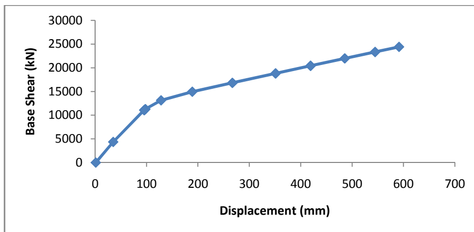
Gambar 12. Kurva Kapasitas Pada Struktur Dengan 40 % Dinding Pengisi Pada Lantai Dasar.
