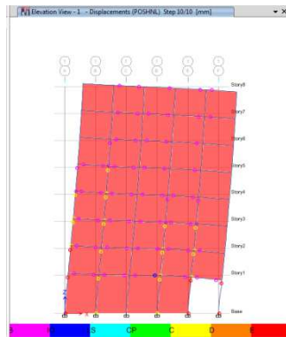
Gambar 15 Hasil Analisis Pushover Pada Struktur Gedung Dengan 80% Dinding Pengisi
