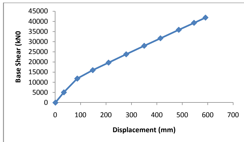
Gambar 14. Kurva Kapasitas Pada Struktur Dengan 60 % Dinding Pengisi Pada Lantai Dasar.
