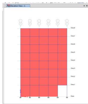
Gambar 5. Struktur Dengan 80% Dinding Pengisi Pada Lantai Dasar
