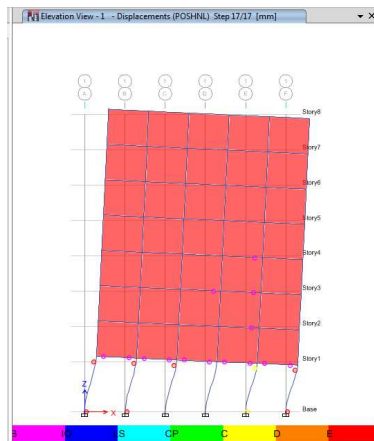
Gambar 7. Hasil Analisis Pushover Pada Struktur Gedung Tanpa Dinding Pengisi
