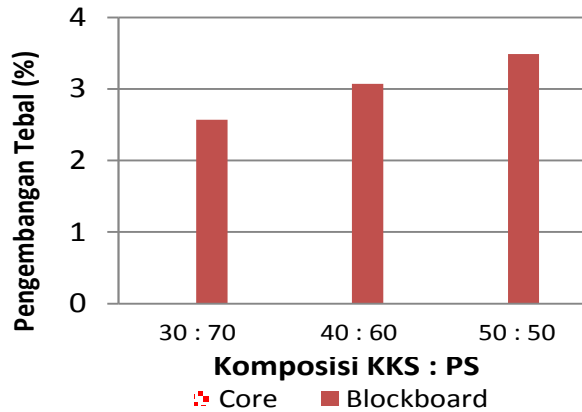
Gambar 7. Pengembangan Tebal Block Board
