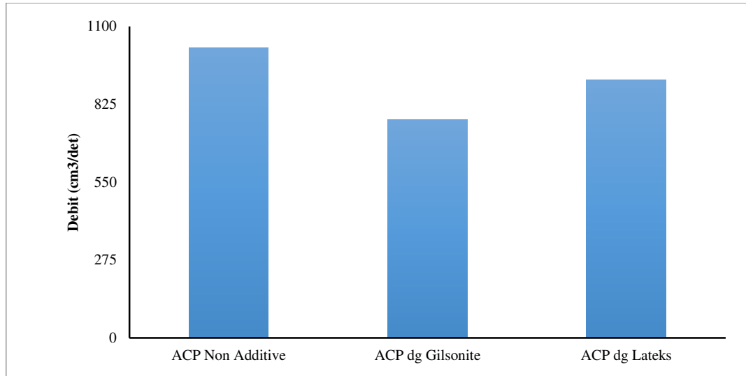
Gambar 2 Perbandingan Nilai Kemampuan Permeabilitas Campuran Beraspal Porus Dengan dan Tanpa Aditif
