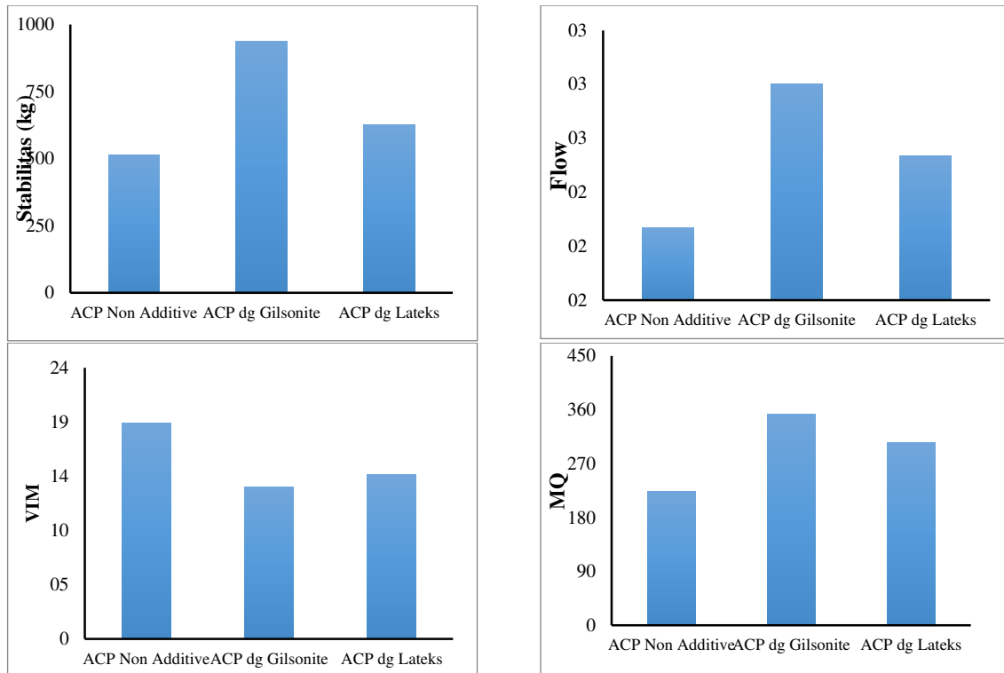
Gambar 1 Perbandingan Nilai Parameter Marshal Campuran Beraspal Porus Dengan dan Tanpa Aditif
