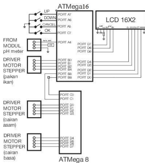
Gambar 1. Blok diagram sistem alat pemberi pakan ikan dan pengontrol PH otomatis
