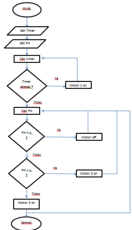
Gambar 2. Diagram Alir Kerja Sistem
