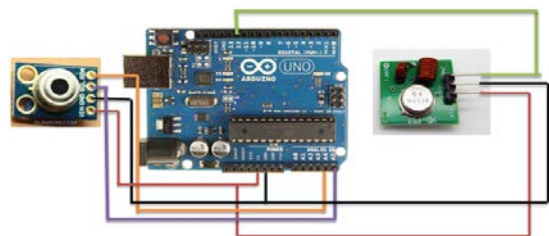
Gambar 8 Blok Rangkaian I
