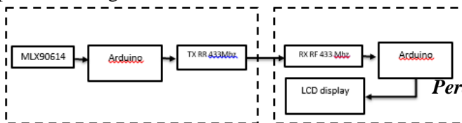
Gambar 5 Diagram blok sistem
