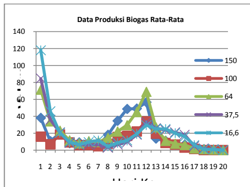
Gambar 4.4 Produksi Biogas Rata-Rata Tanpa Proses Penghalusan (Cacah) dan Variasi Pengenceran
