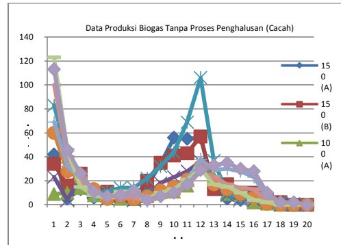
Gambar 4.3 Produksi Biogas Tanpa Proses Penghalusan (Cacah) dan Variasi Pengenceran
