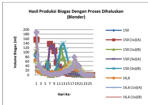
Gambar 4.7 Produksi Biogas Dengan Proses Penghalusan (Blender), Variasi Pengenceran dan Pengadukan
