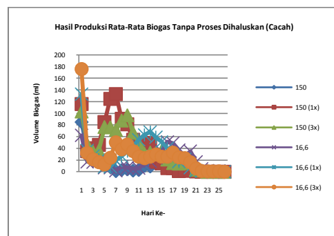
Gambar 4.10 Produksi Biogas Rata-Rata Tanpa Proses Penghalusan (Cacah), Variasi Pengenceran dan Pengadukan
