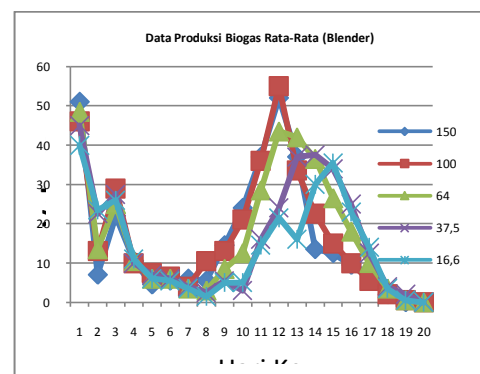
Gambar 4.2 Produksi Biogas Rata-Rata Dengan Proses Penghalusan (Blender) dan Variasi Pengenceran
