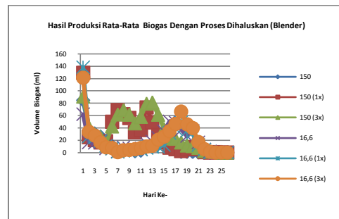
Gambar 4.8 Produksi Biogas Rata-Rata Dengan Proses Penghalusan (Blender), Variasi Pengenceran dan Pengadukan
