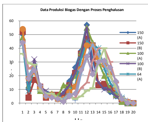
Gambar 4.1 Produksi Biogas Dengan Proses Penghalusan (Blender) dan Variasi Pengenceran
