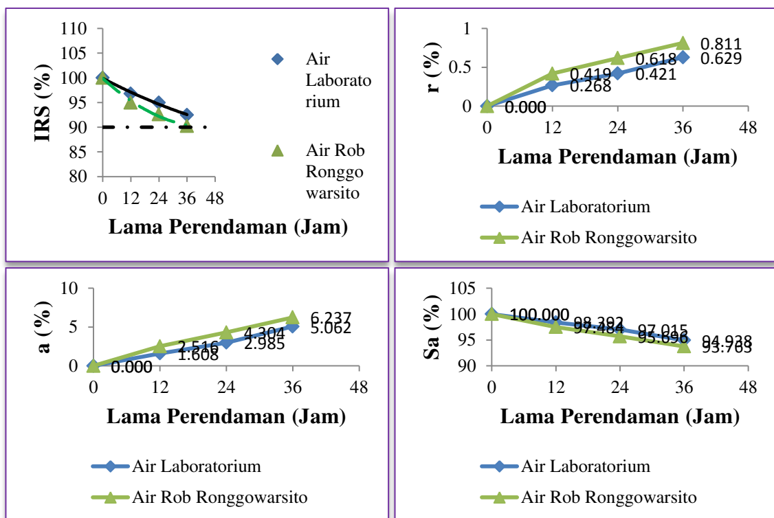
Gambar 4. Hubungan Nilai IRS, IDP, dan IDK dan Waktu Perendaman dengan Pola Berkala
