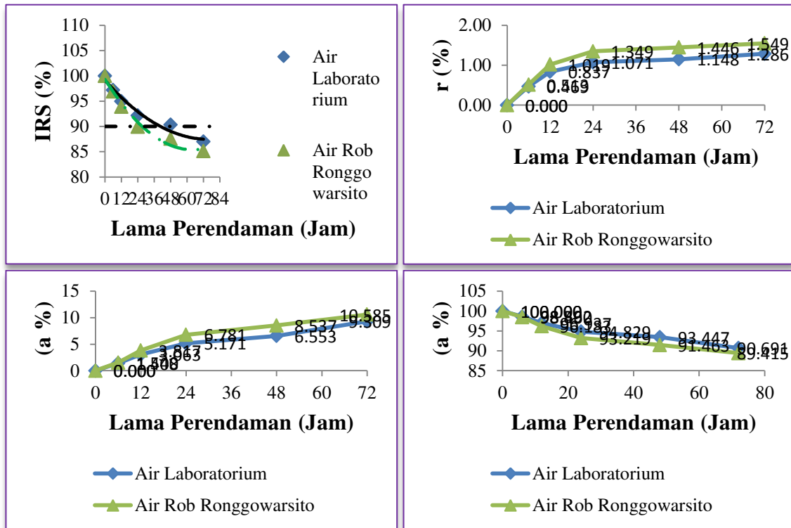
Gambar 3. Hubungan Nilai IRS, IDP, dan IDK dan Waktu Perendaman dengan Pola Menerus
