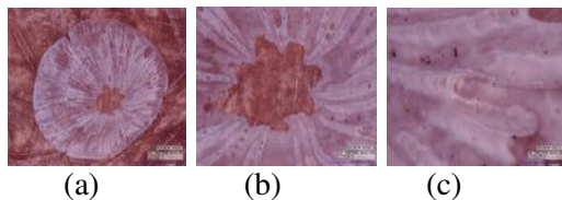
Gambar 14. Morphology sampel pelat blister bercak putih dengan perbesaran 50X (a), 150X (b) dan 350X (c)
