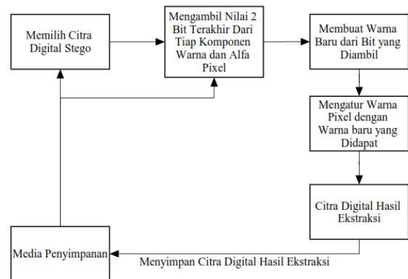
Gambar 3. Diagram blok proses ekstraksi citra digital pesan
