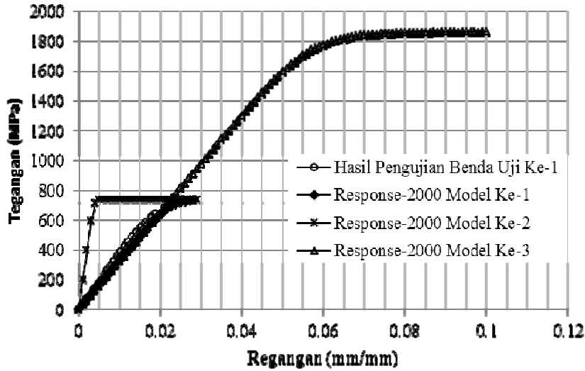
Gambar 8. Perbandingan hubungan tegangan-regangan wire rope hasil pengujian dan pemodelan
