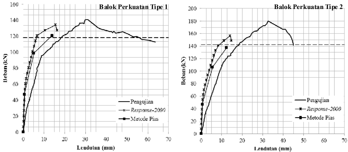
Gambar 10. Perbandingan hubungan beban-lendutan balok perkuatan
