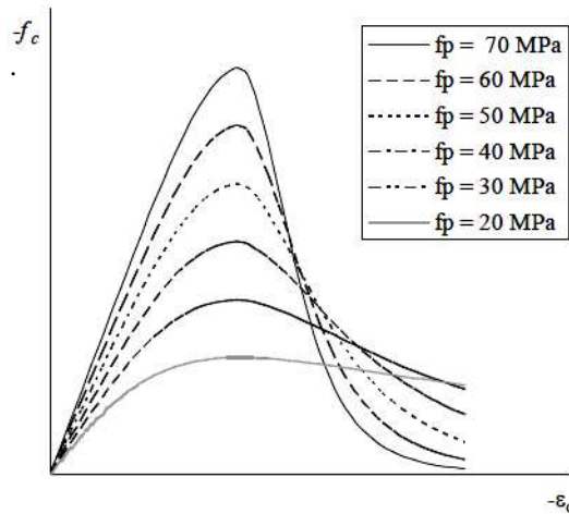
Gambar 4. Hubungan tegangan-geganan beton Model Popovics (Bentz, 2000)
