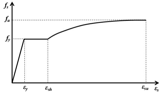
Gambar 5. Hubungan tegangan-regangan baja Model Parabolik
