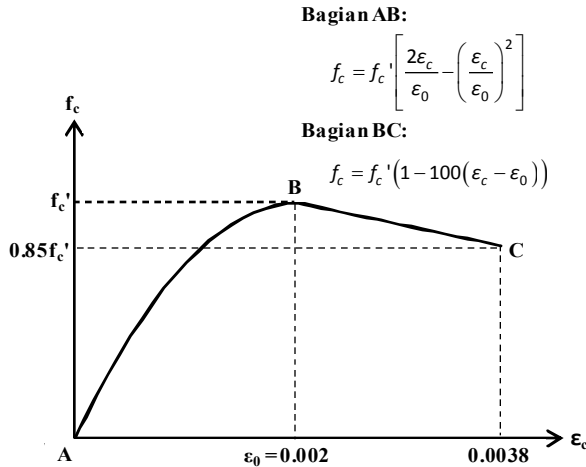
Gambar 7. Hubungan tegangan-regangan beton Model Hognestaad
