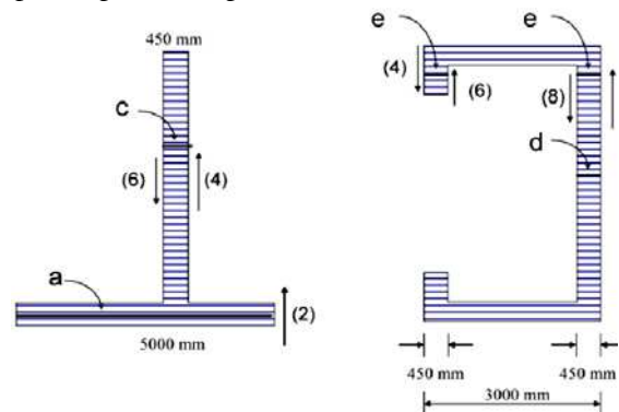
Gambar 2. Contoh pembagian pias penampang elemen (Lam dkk, 2011)
