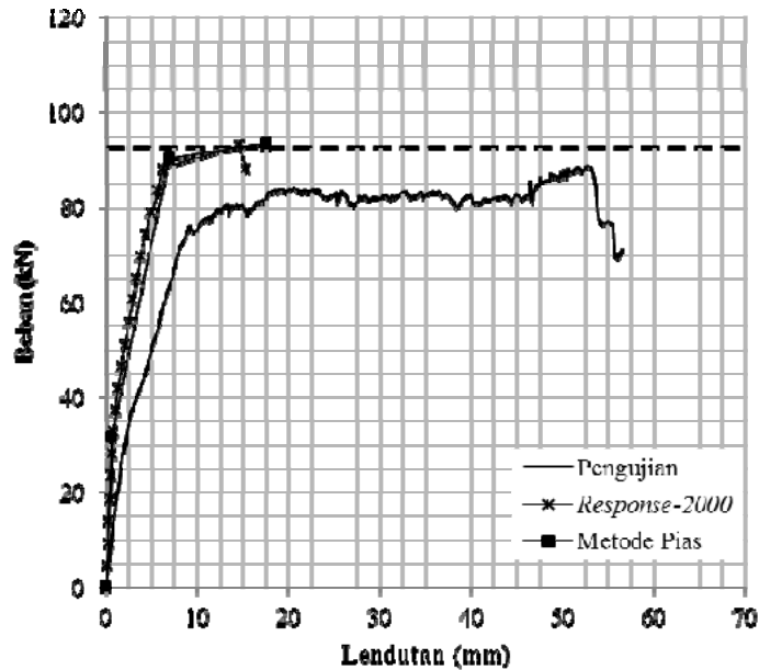
Gambar 9. Perbandingan hubungan beban-lendutan balok kontrol
