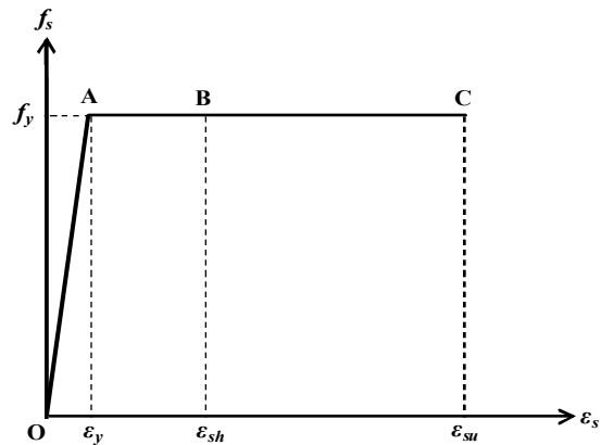
Gambar 6. Hubungan tegangan-regangan baja Model Bilinear (Park dan Pauly, 1975)
