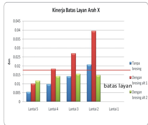
Gambar 5.14. Perbandingan kinerja batas layan arah X struktur tanpa dan dengan bresing
