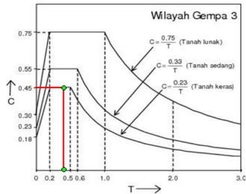
Gambar 5.10. Respons spektrum gempa wilayah gempa 3
