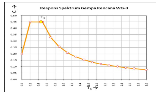
Gambar 5.11. Respon spektrum gempa rencana
