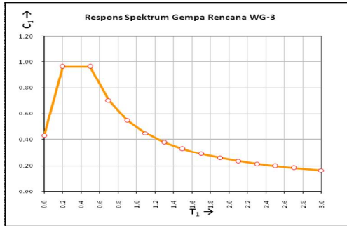
Gambar 5.12. Respon spektrum gempa rencana terkorreksi
