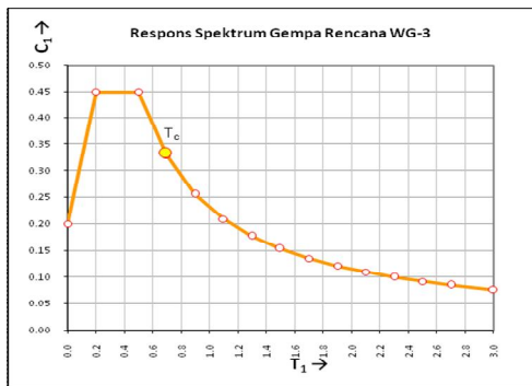
Gambar 5.7. Respon spektrum gempa rencana terkoreksi
