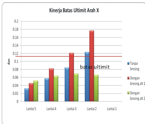
Gambar 5.16. Perbandingan kinerja batas ultimit arah X struktur tanpa dan dengan bresing
