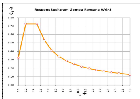
Gambar 5.6. Respon spektrum gempa Rencana
