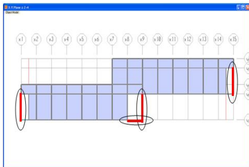
Gambar 5.13. Lokasi penambahan bresing alternatif 2
