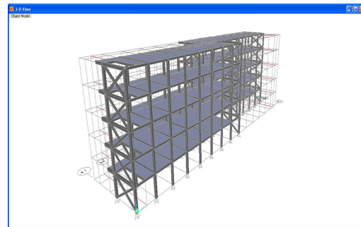
Gambar 4.2. Model Struktur dengan B्रेसing X
