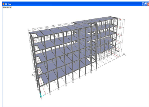
Gambar 4.1. Model Struktur Dimensi
