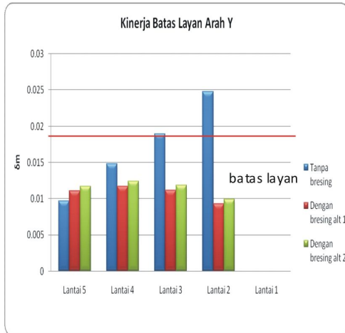
Gambar 5.15. Perbandingan kinerja batas layan arah Y struktur tanpa dan dengan bresing
