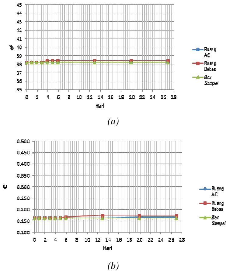
Gambar 7. Grafik Perubahan Nilai Sudut Geser Dalam (a) dan Kohesi (b) sampel Namosain
