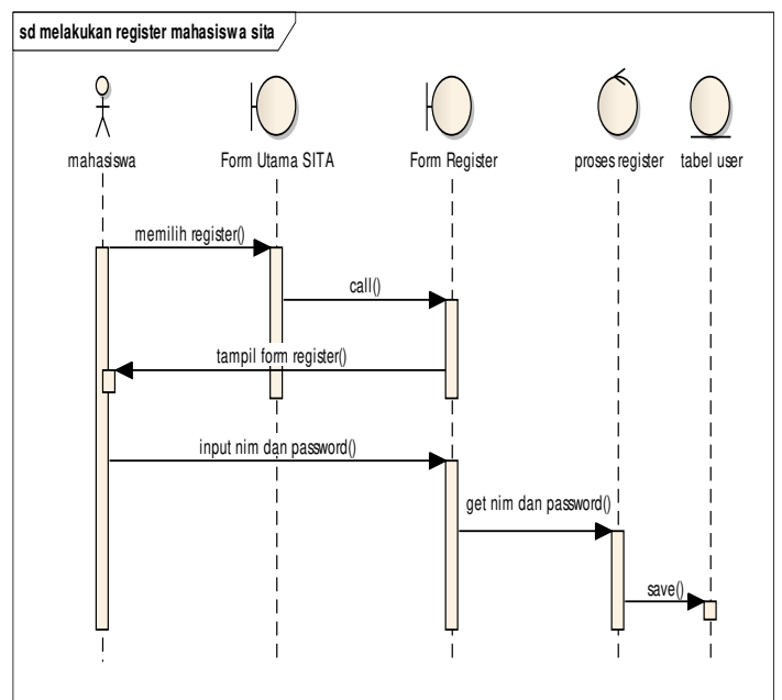
Gambar 5. Sequence Diagram Melakukan Register
