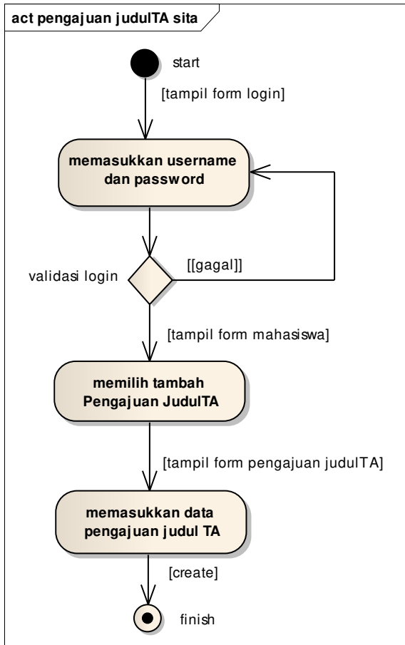
Gambar 3. Activity Diagram Pengajuan JudulTA Mahasiswa
