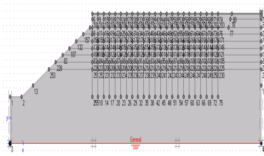
Gambar 14. Pendefinisian Kondisi Awal Tanah pada Perangkat Lunak Plaxis.
